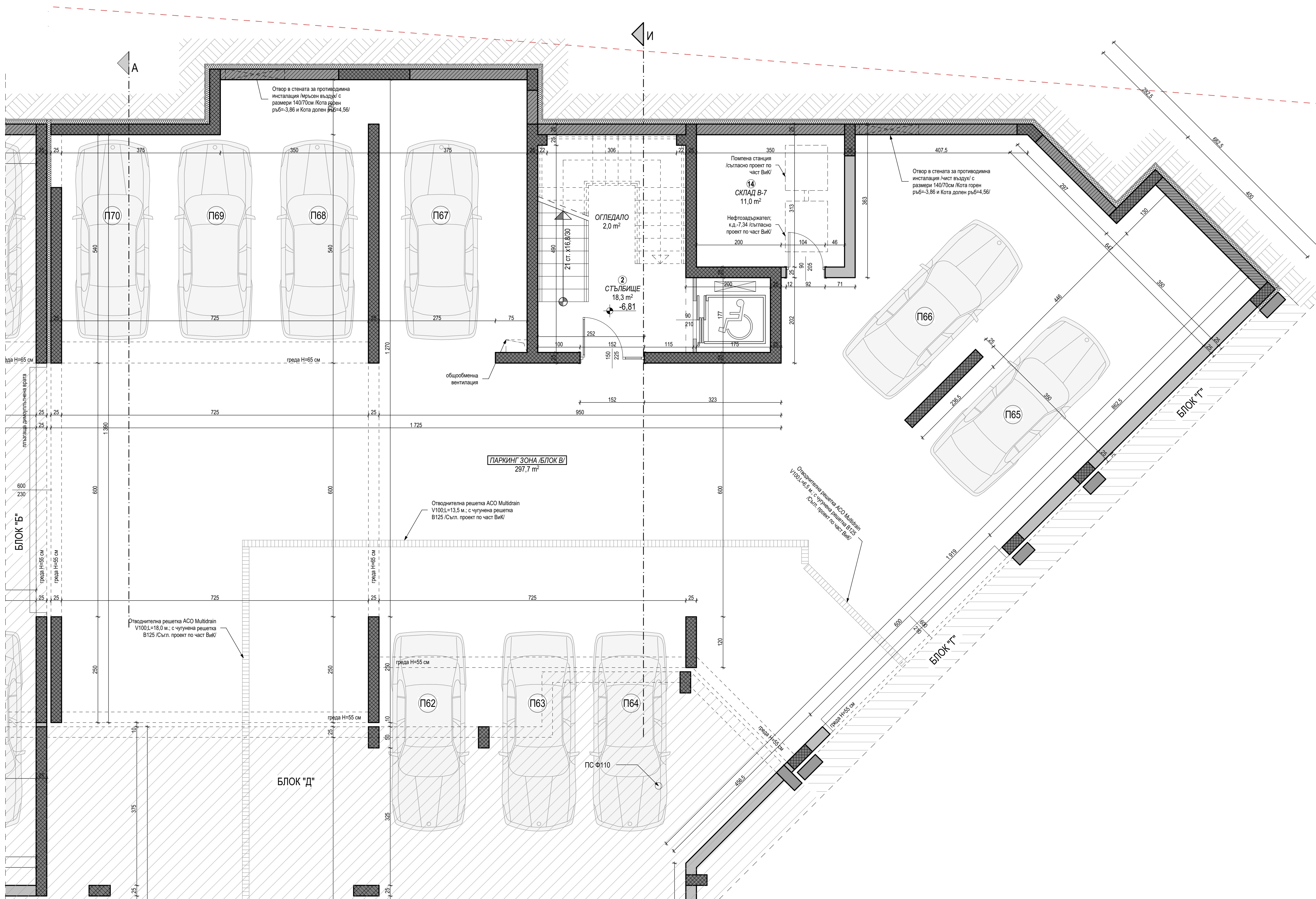
Разпределение на кота -6,81 /Блок В/ М 1:50
